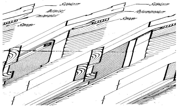
Tetting av fugens utside med forskjellige materialer
