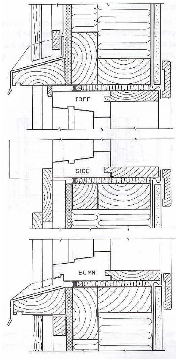
Vindu i trevegg
