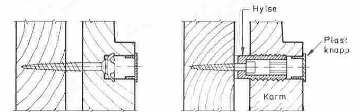
Innfesting med feste- og justeringshylser
