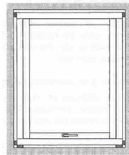
Plassering av bæreklosser og kiler
