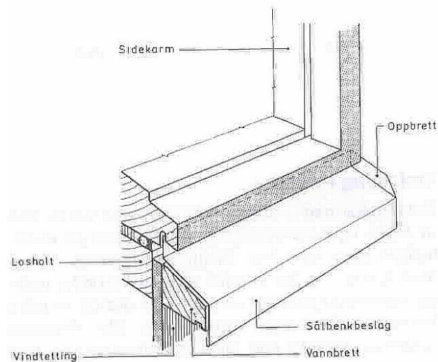
Plassering av sålbenksbeslag
