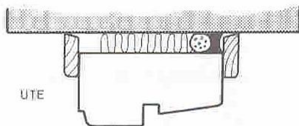
Ytre tetting sløyfet
